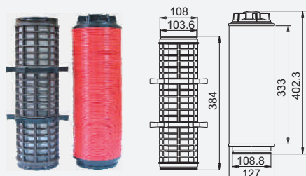
3481-3431 Cartridge for Proteas / Proteas-Spin Εσωτερικά στοιχεία φίλτρου Protea / Proteas-Spin
