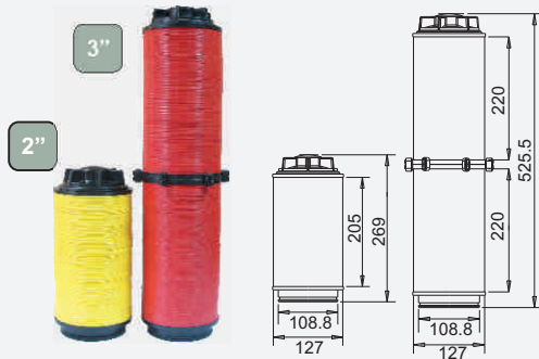
3482 Cartridge for Typhoon Εσωτερικά στοιχεία φίλτρου Typhoon
