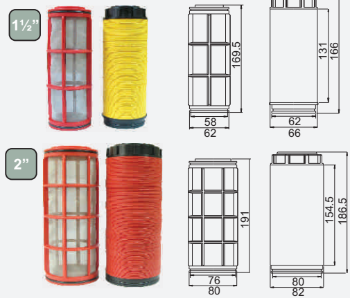
3481-3484-4481 Cartridge for In-Line Filters 1 1/2" & 2" Εσωτερικά στοιχεία Φίλτρων Γραμμής 1 1/2" & 2"
