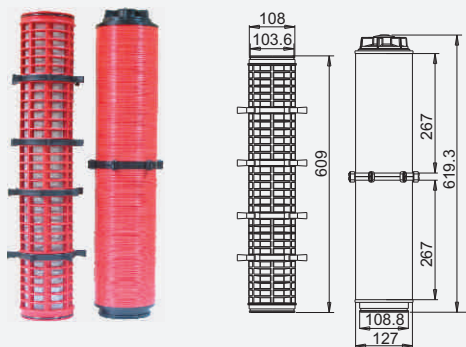
3481-3431 Cartridge for Proteas / Proteas-Spin Εσωτερικά στοιχεία φίλτρου Protea / Proteas-Spin
