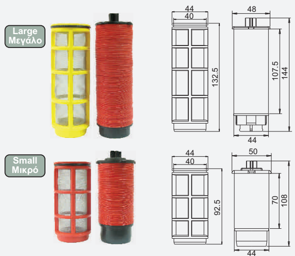
3481-3482 Cartridge for In-Line Small / Large Filters Εσωτερικά στοιχεία για Φίλτρο Μικρό / Μεγάλο
