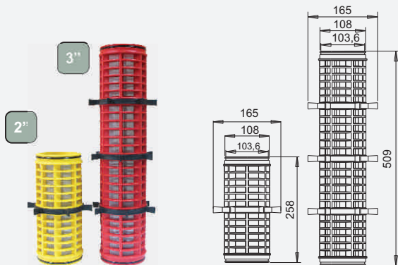
3481 Cartridge for Hydro / Hydro-Spin Εσωτερικά στοιχεία φίλτρου Hydro / Hydro-Spin
