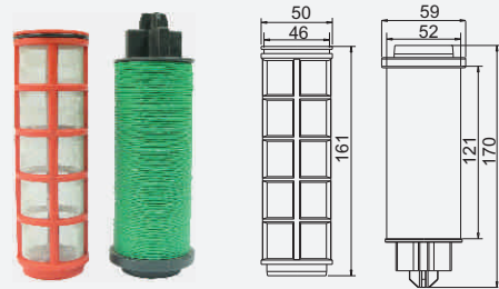
3481-4482 Cartridge for Filter Special Εσωτερικά στοιχεία φίλτρου Special
